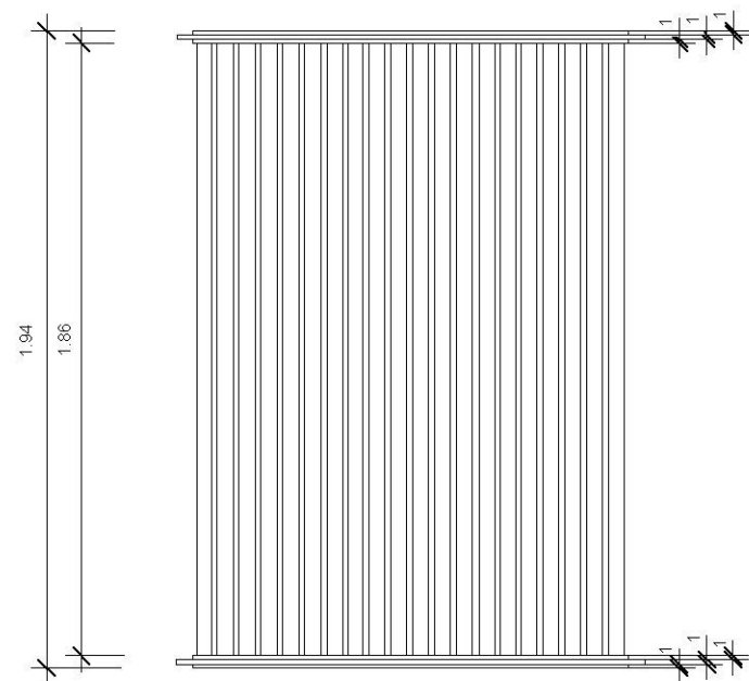
Schachbanktyp ohne Lehne mit Schubladen 1:25
