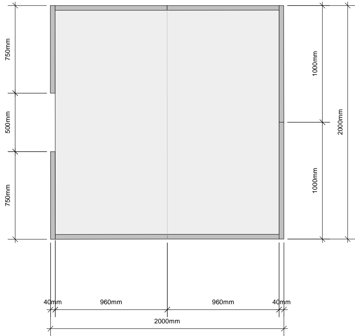
Grundriss
